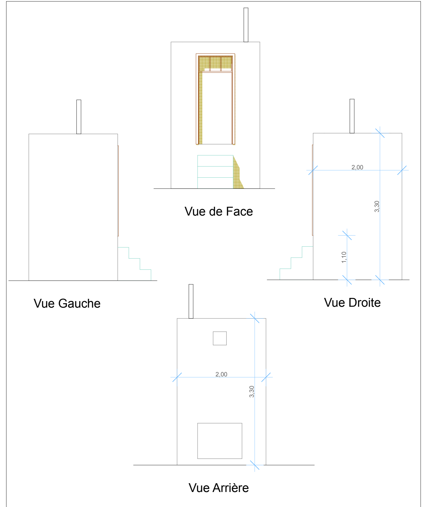
Façades Latrine Simple
