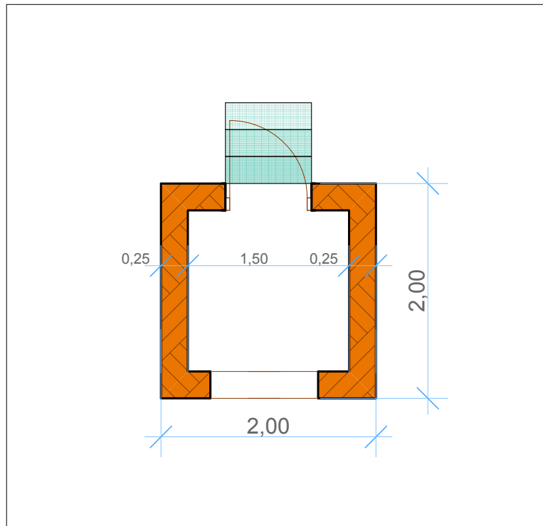
Plan Latrine Simple
